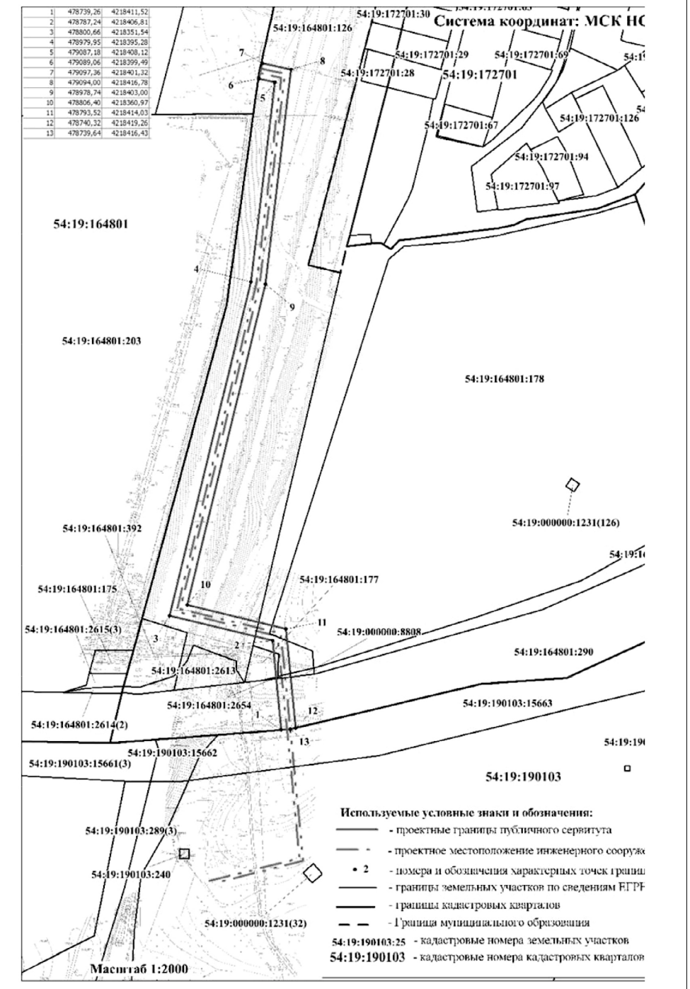
Схема расположения границ публичного сервитута устанавливается для использования земельных участков строительства шпурной ливневой канализации от ЦКП «СКИФ» до централизованной системы водоотведения сточных вод в районе р.Ноздриха в р.п. Кольцово Новосибирской области
